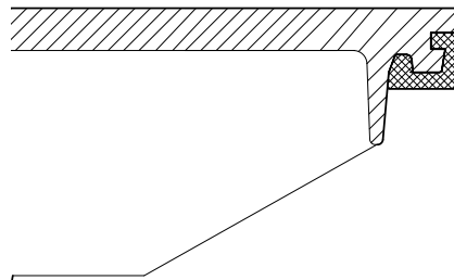
Snittegning av BALDER lokk med påstøpt pakning
